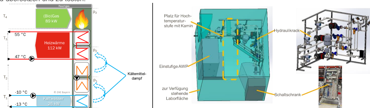
Prozesskonzept & Aufstellungsplanung der Laboranlage
